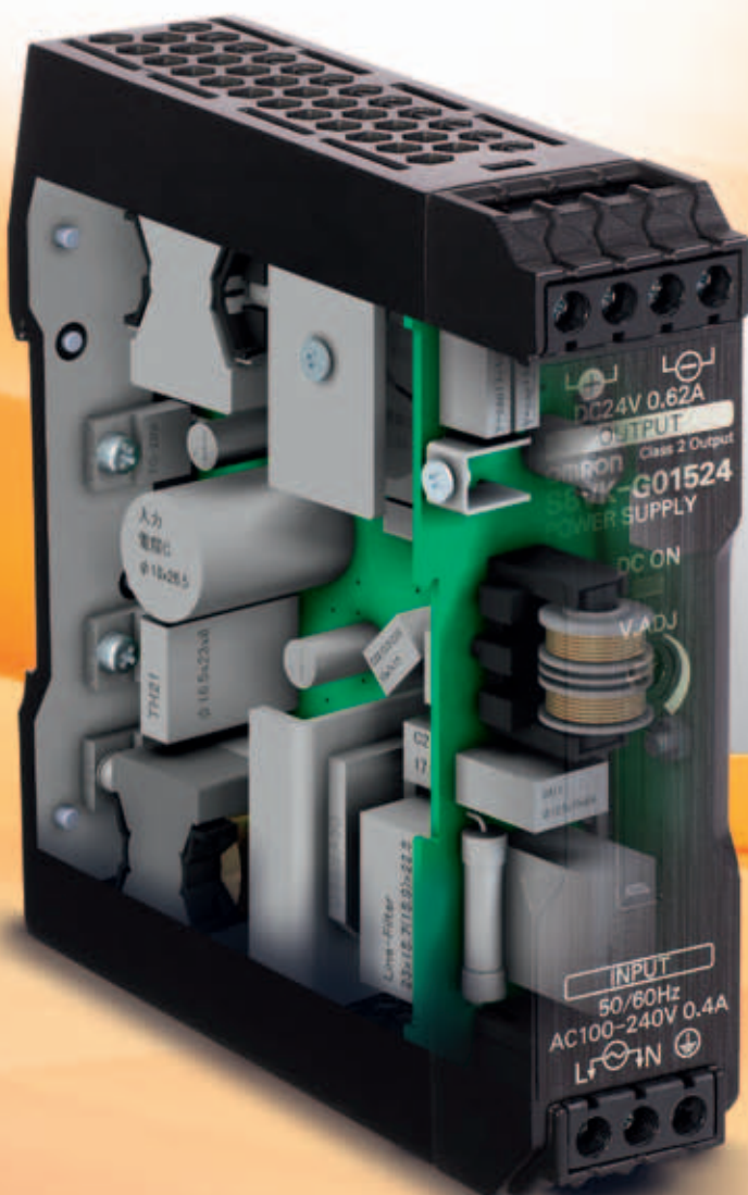
Zobrazení součástek
